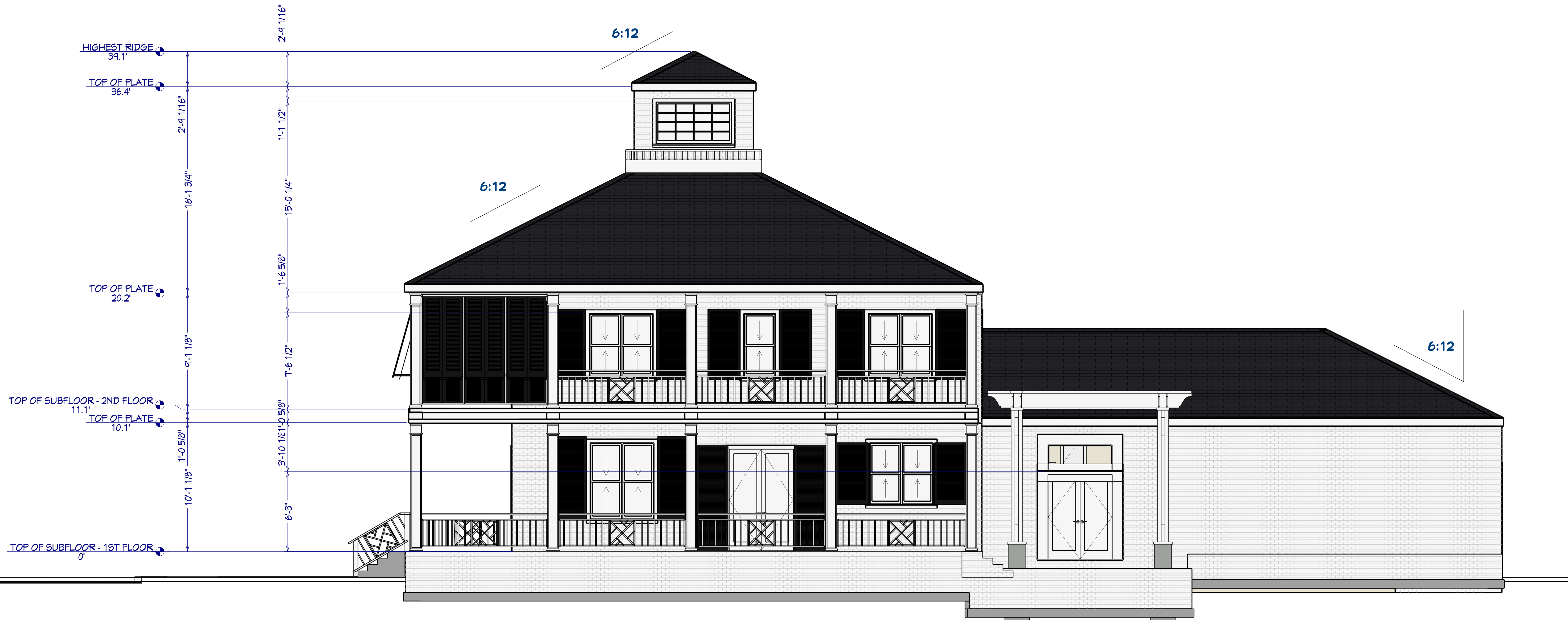
Right Elevation
