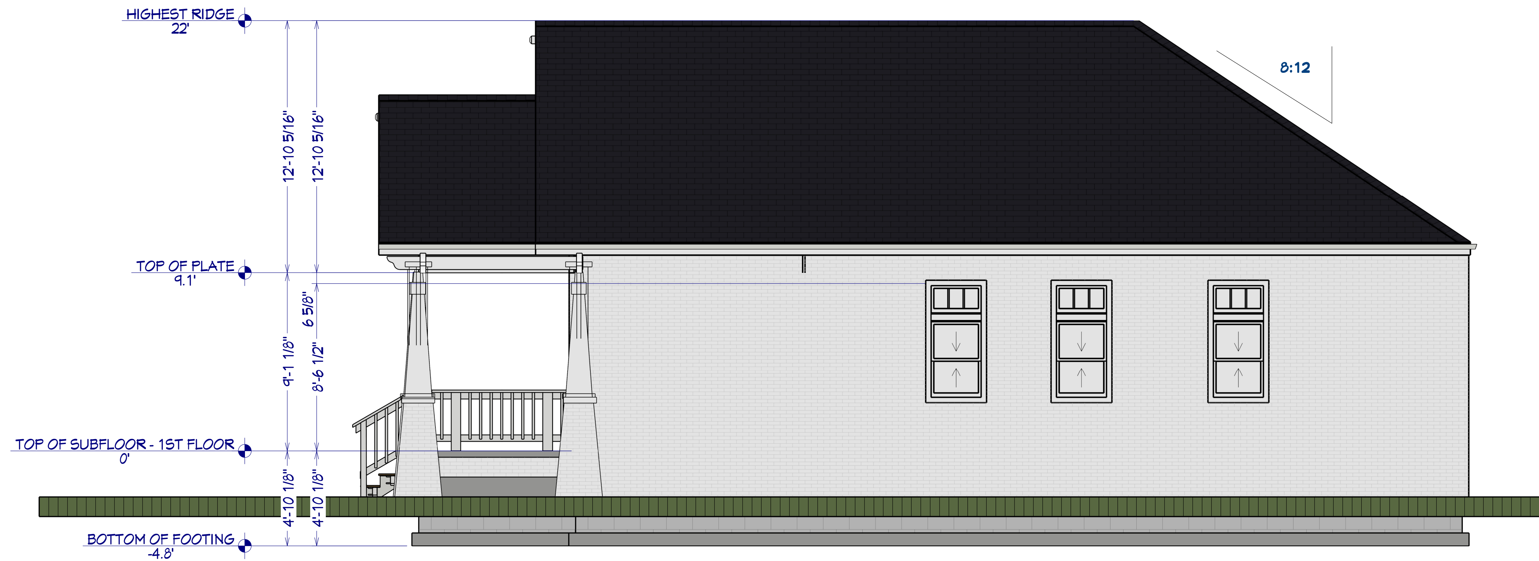
Right Elevation
